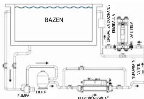
Model s inteligentnom pumpom za doziranje
