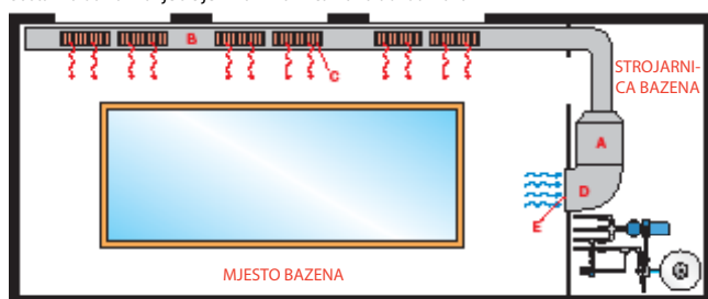
Uređaj za odvlaživanje unutar strojarnice bazena
