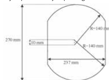
Mjere pozicioniranja rupa za ugradbeni dio
