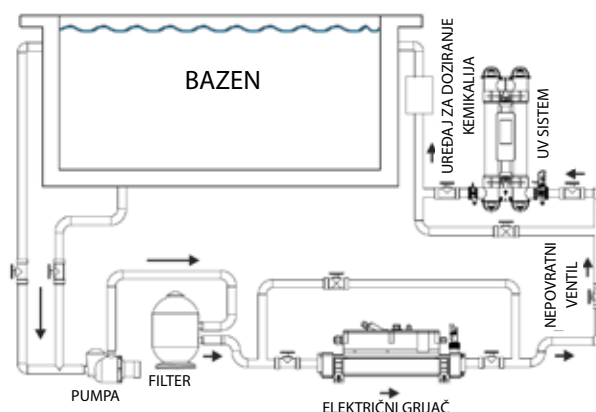
Model s peristaltičkom pumpom
